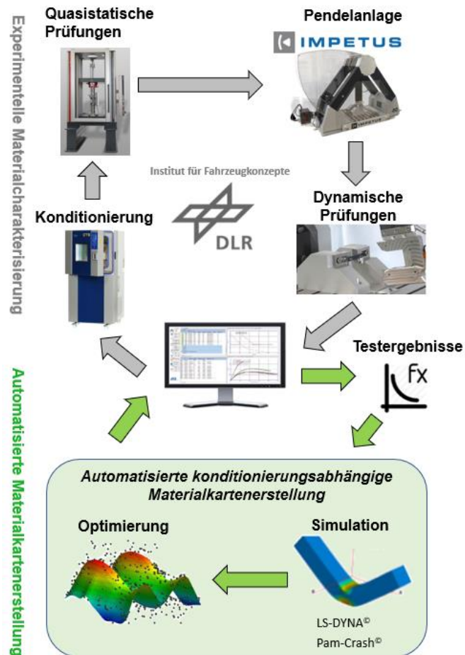
Prozessablauf für die automatisierte Materialkartenableitung
