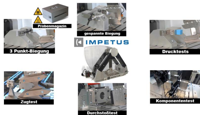
Verfügbare Testaufbauten für die dynamische Materialcharakterisierung
